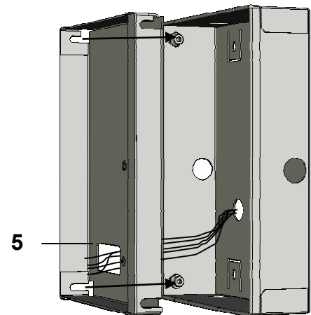
Einbaurahmen
